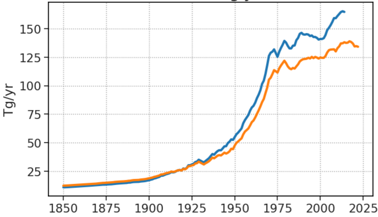
NMVOC Tg/yr
