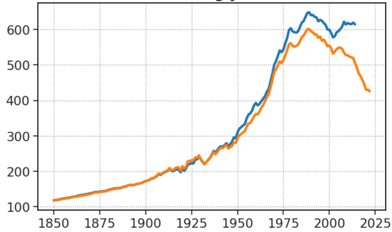
CO2 Tg/yr
