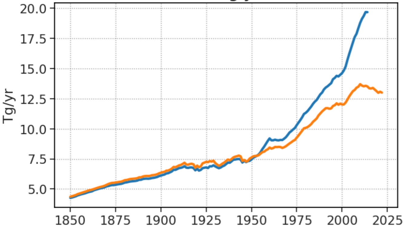
NMVOC Tg/yr
