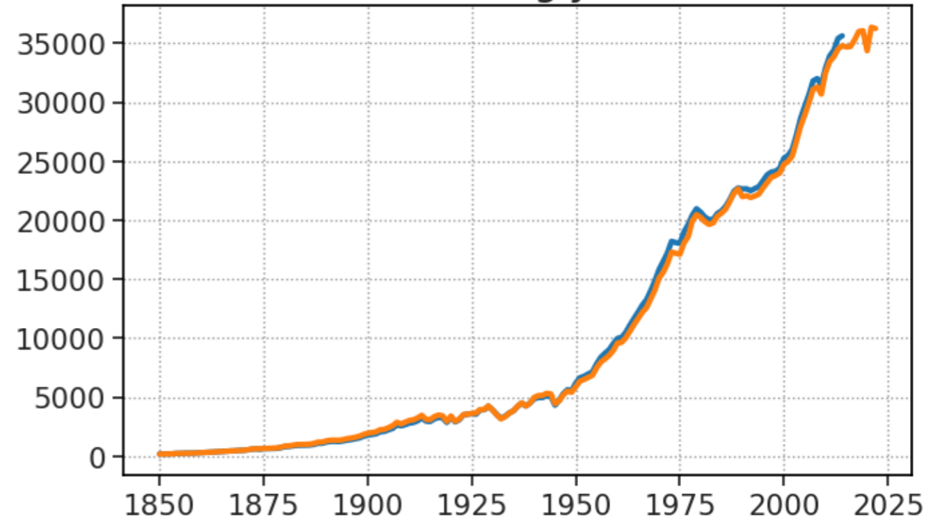
CO2 Tg/yr
