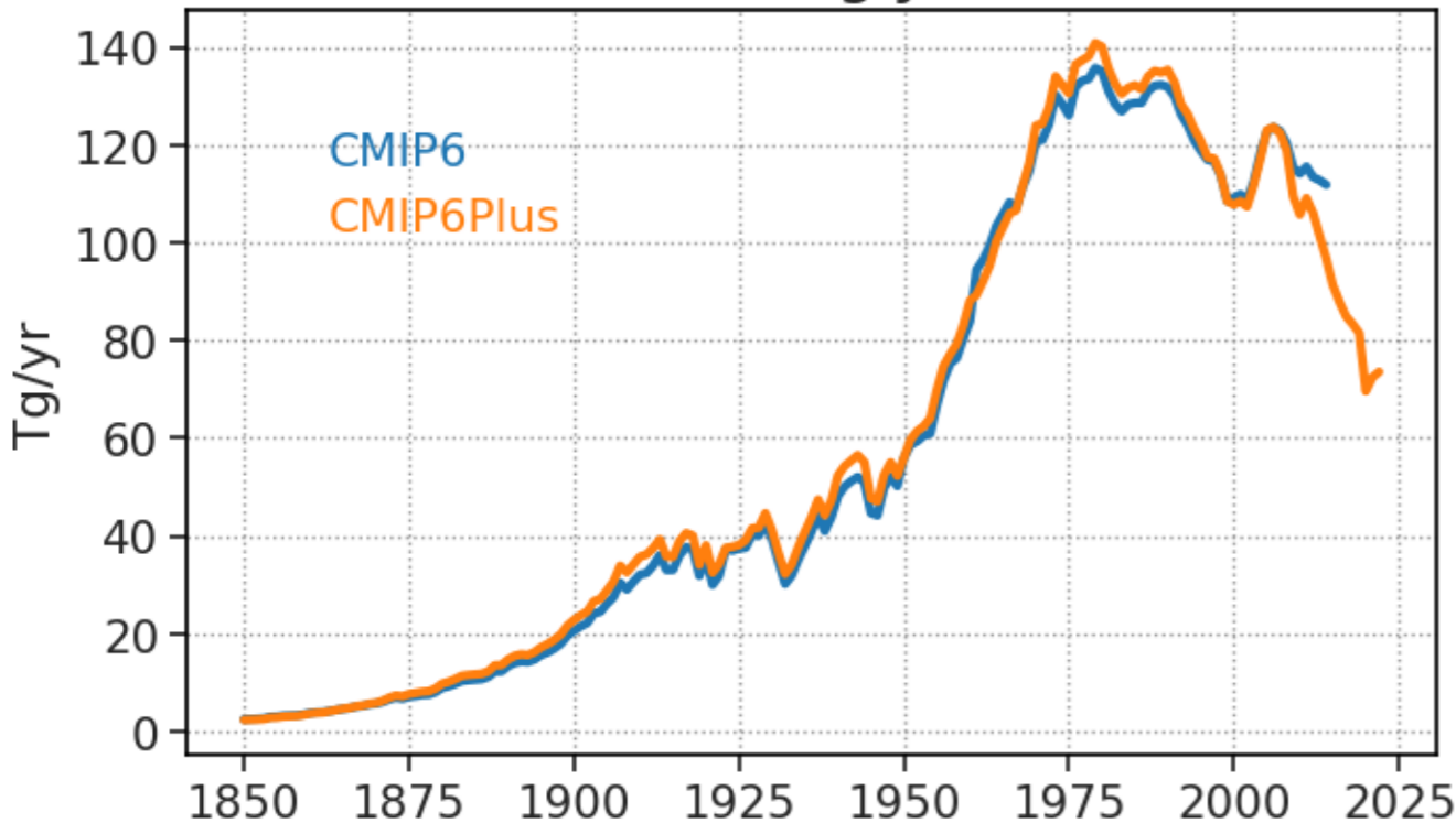
NH3 Tg/yr
